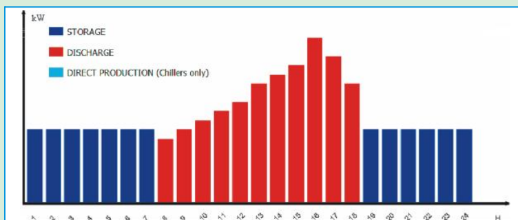
Стратегия полного использования аккумулятора холода
