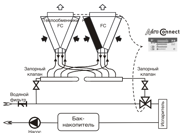
Схема модуля естественного охлаждения
